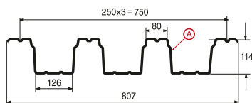
Профилированный лист Н-114x750-А
