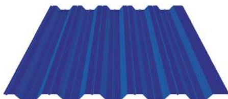
Профилированный лист МП-20х1100-R Толщина материала 0.4 - 0.8 мм
