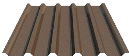
Профилированный лист НС-35х1000-A Толщина материала 0.45 - 0.9 мм
